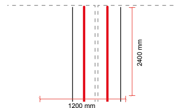
Doble cordón en montante o pie derecho con encuentro de placas
